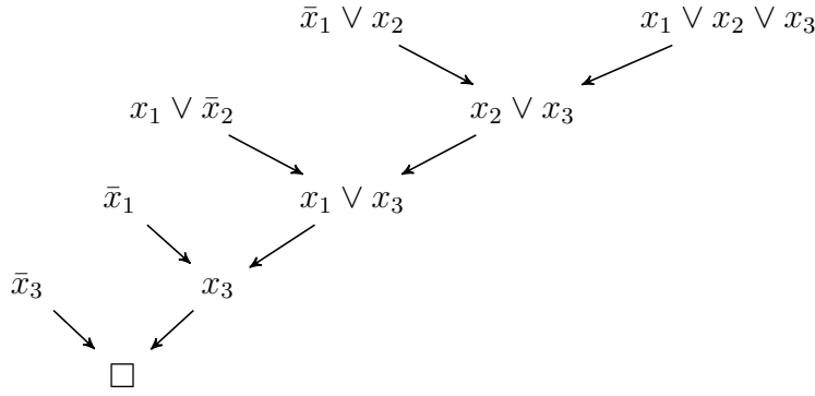
Figura 2.1: Prueba de resolución
