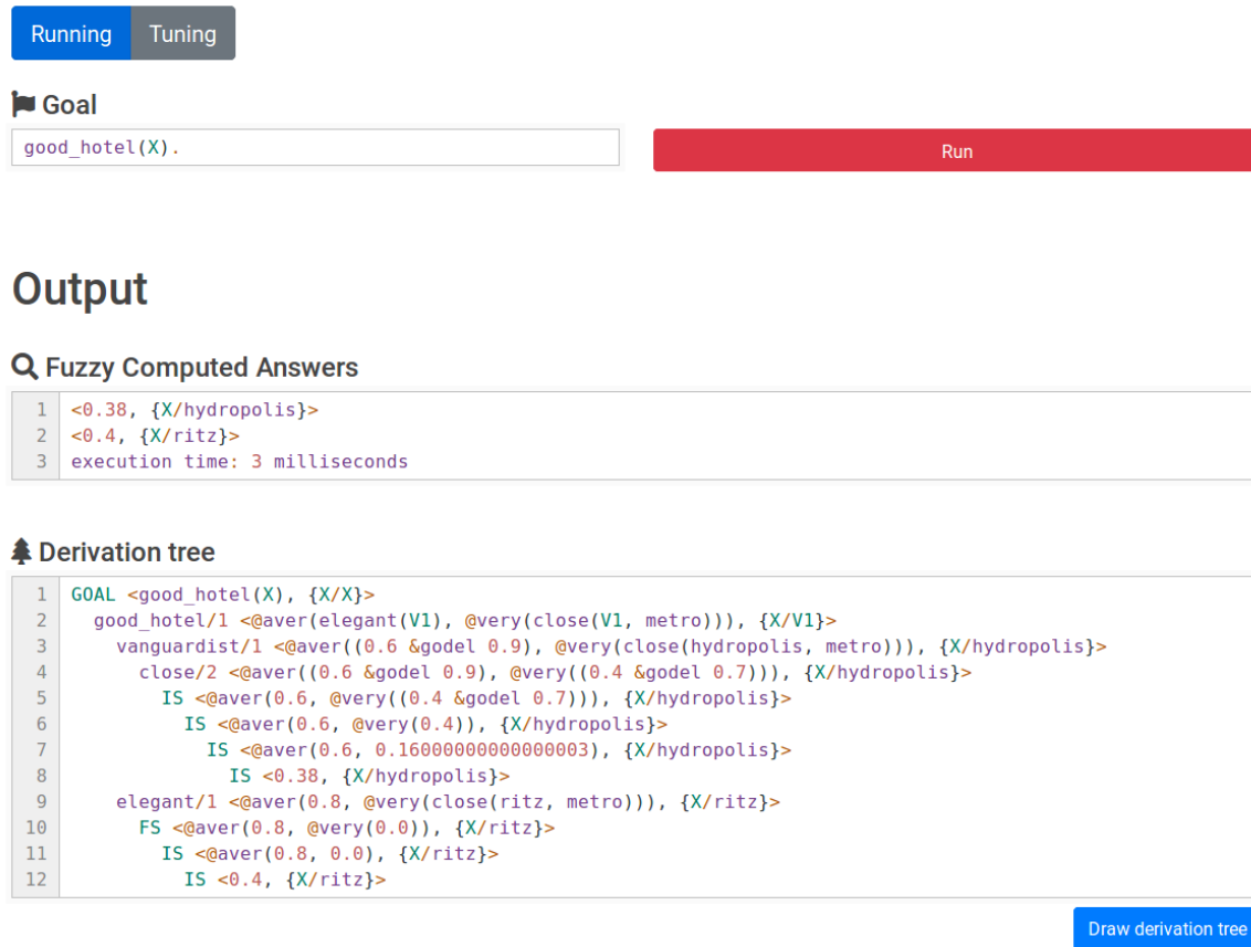
Figura 2.6: Captura de pantalla de la herramienta FASILL online tras ejecutar un objetivo
